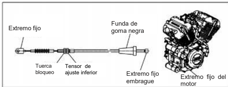
Figura 22 Embrague
