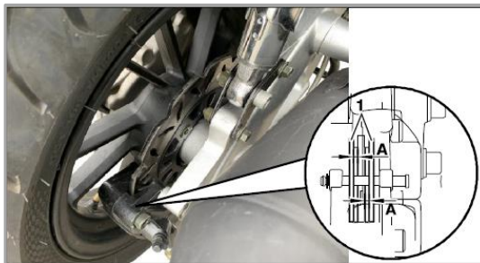
Pastilha de travão traseira
