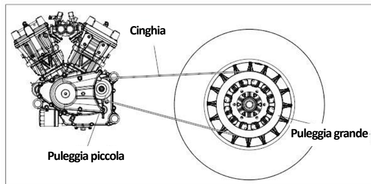
Figura 21 Trasmissione a cinghia
