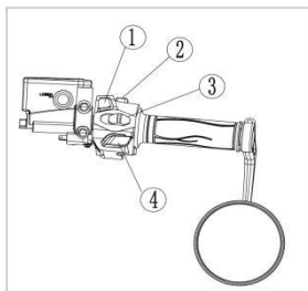
Fig.6 Combinación de interruptores derecha
