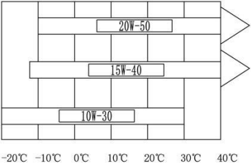
Abb.15 Schmierölkontrolle
