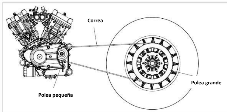
Figura 21 Transmisión por correa
