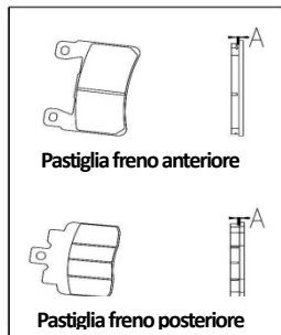
Figura 29 Controllo della guarnizione d'attrito freno
