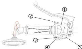
Abb.7 Linke Schalterkombination
