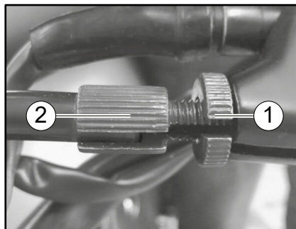
1. Frette embrayage 2. Vis embrayage
