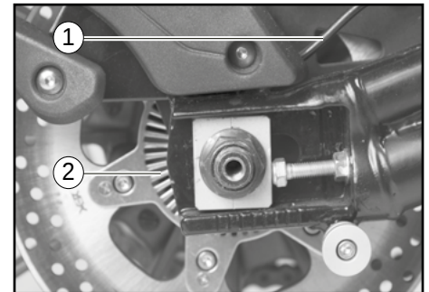
1. Hinterrad-Sensor 2. Sensor-Rotor hinten
