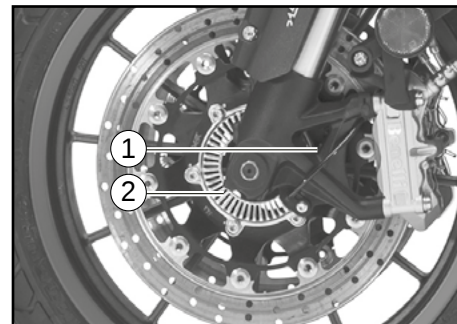
1. Sensore ruota anteriore 2. Ruota fonica ruota anteriore
