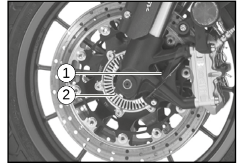
1. Vorderrad-Sensor 2. Sensor-Rotor vorn
