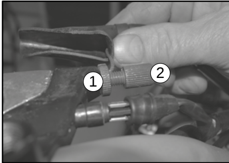
1. Ghiera frizione 2. Vite frizione
