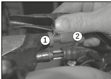
1. Abrazadera del embrague 2. Tornillo embrague
