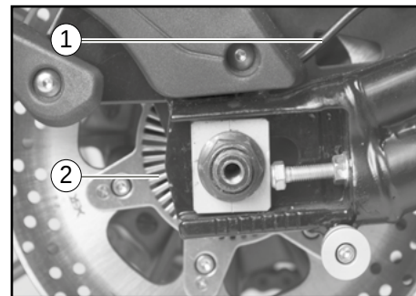
1. Sensore ruota posteriore 2. Ruota fonica ruota posteriore
