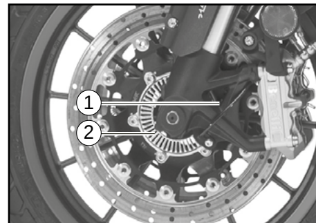
1. Capteur de roue avant 2. Rotor de capteur de roue avant
