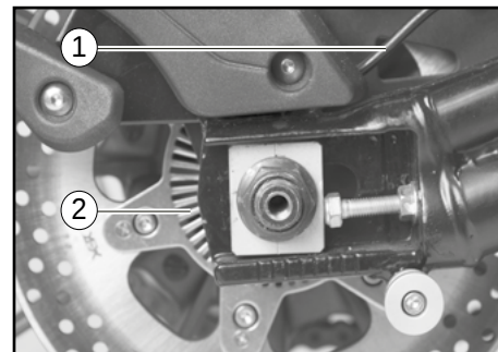
1. Capteur de roue arrière 2. Rotor de capteur de roue arrière
